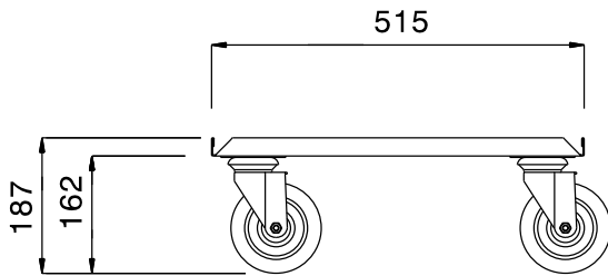
Вид спереди
